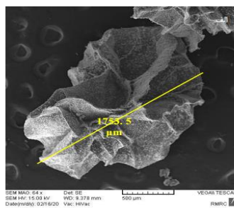
شکل ۵- میکروکپسول‌های ۴ لایه آلژینات کیتوزان (ACAC) بعد از خشک کردن انجمادی
